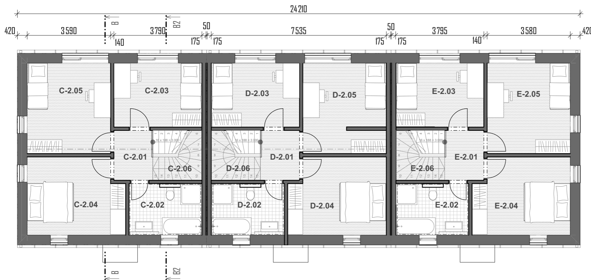
PŮDORYS PODKROVÍ
