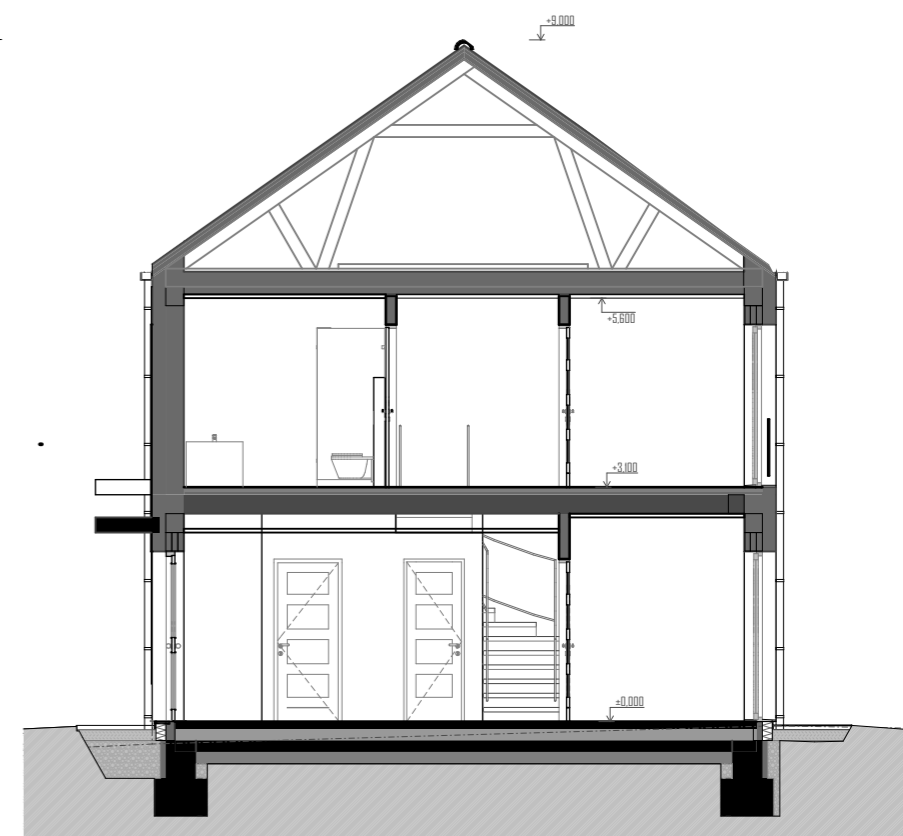
ŘEZ PŘÍČNÝ
